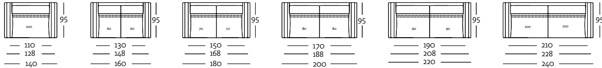
SOB 450/SB 100 SOB 450/SB 120 SOB 450/SB 140 SOB 450/SB 160 SOB 450/SB 180 SOB 450/SB 200
